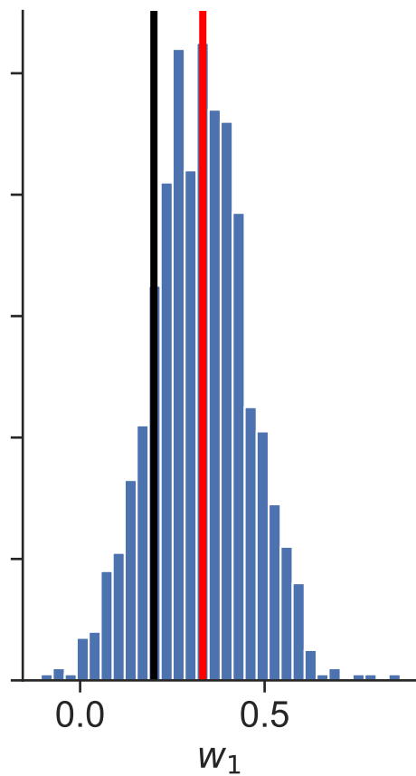
Posterior distributions Dataset 46
