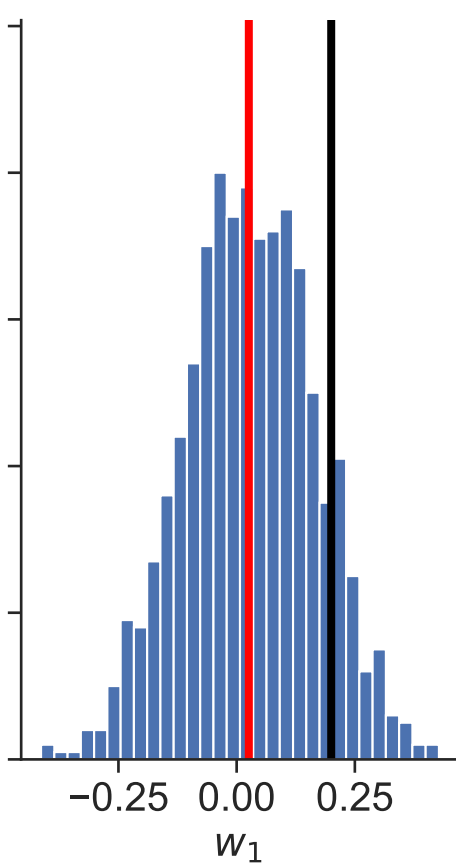
Posterior distributions Dataset 26
